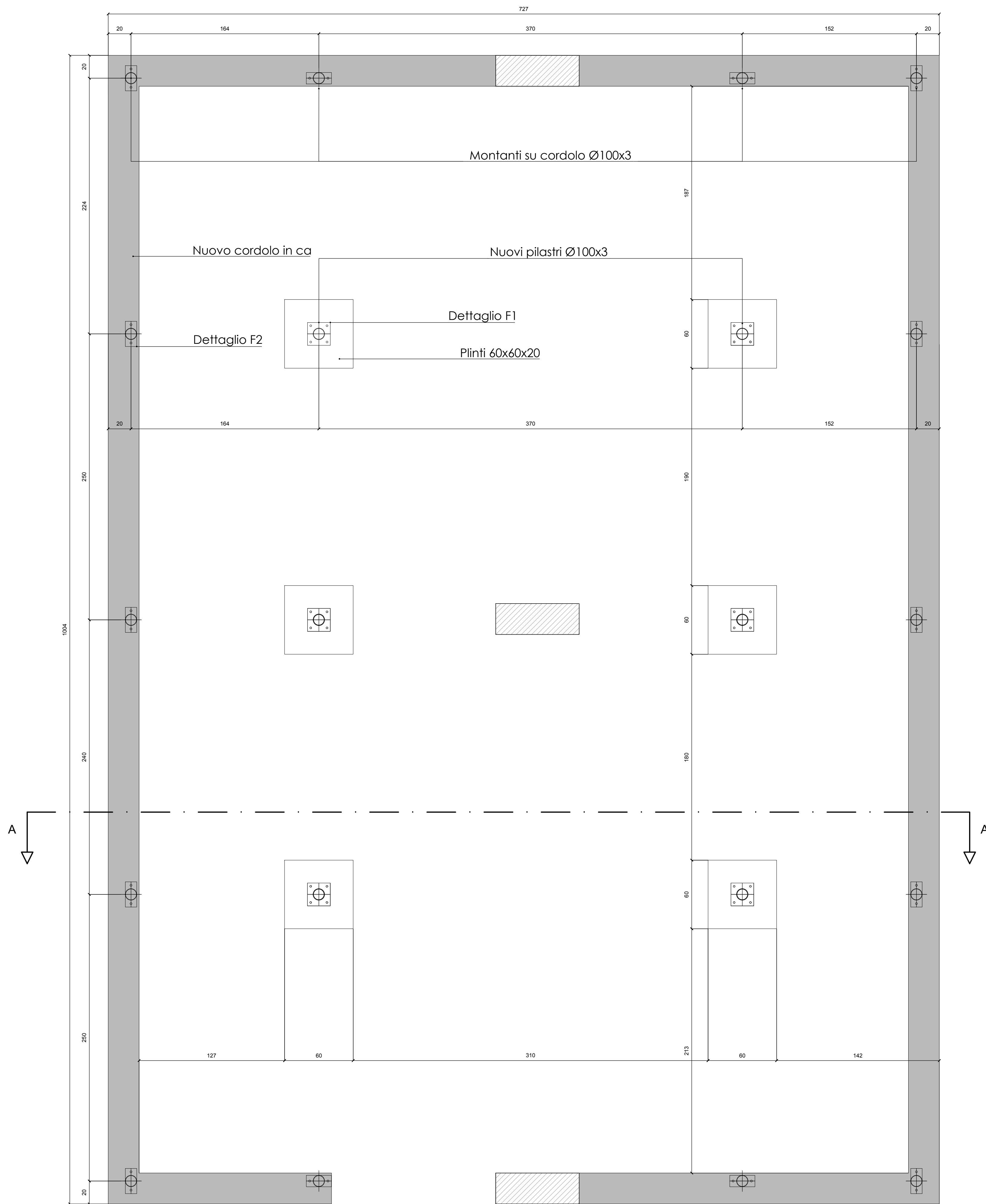
PIANTA FONDAZIONI - SCALA 1:20
