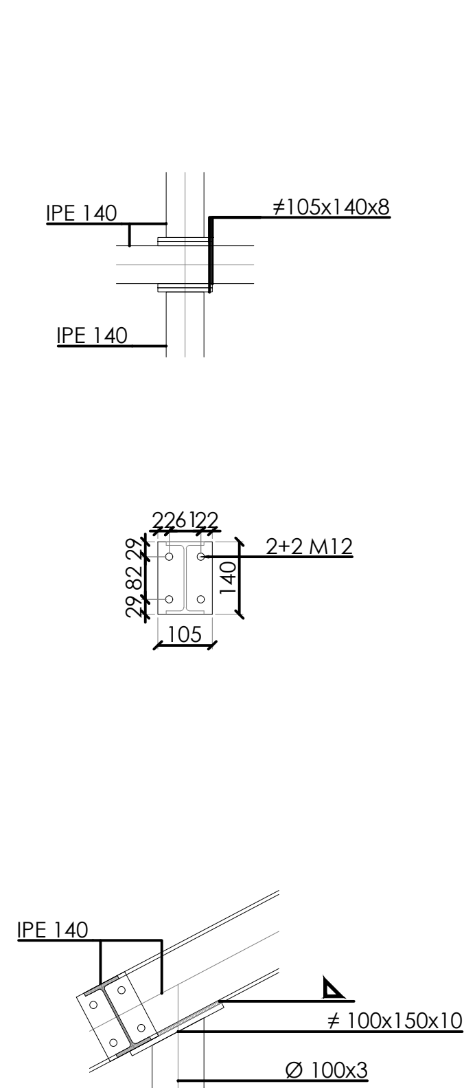
DETTAGLIO 2 - SCALA 1:10
