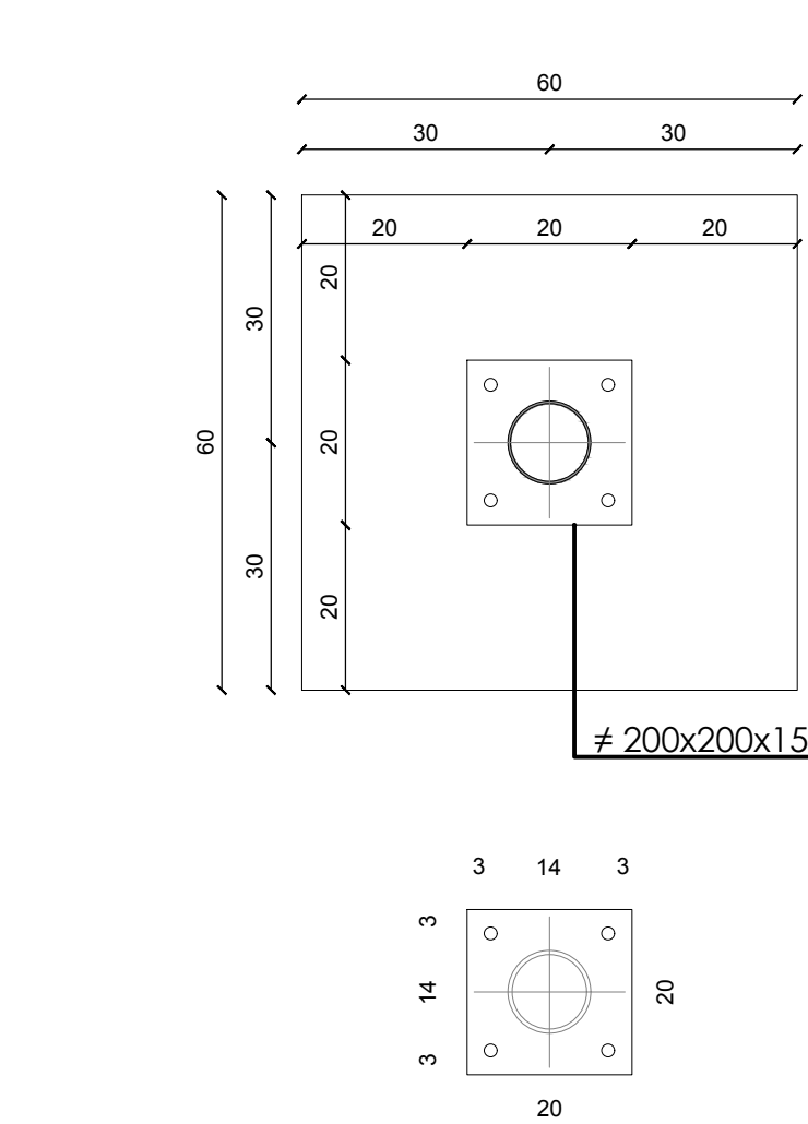
DETTAGLIO F-1 - SCALA 1:10
