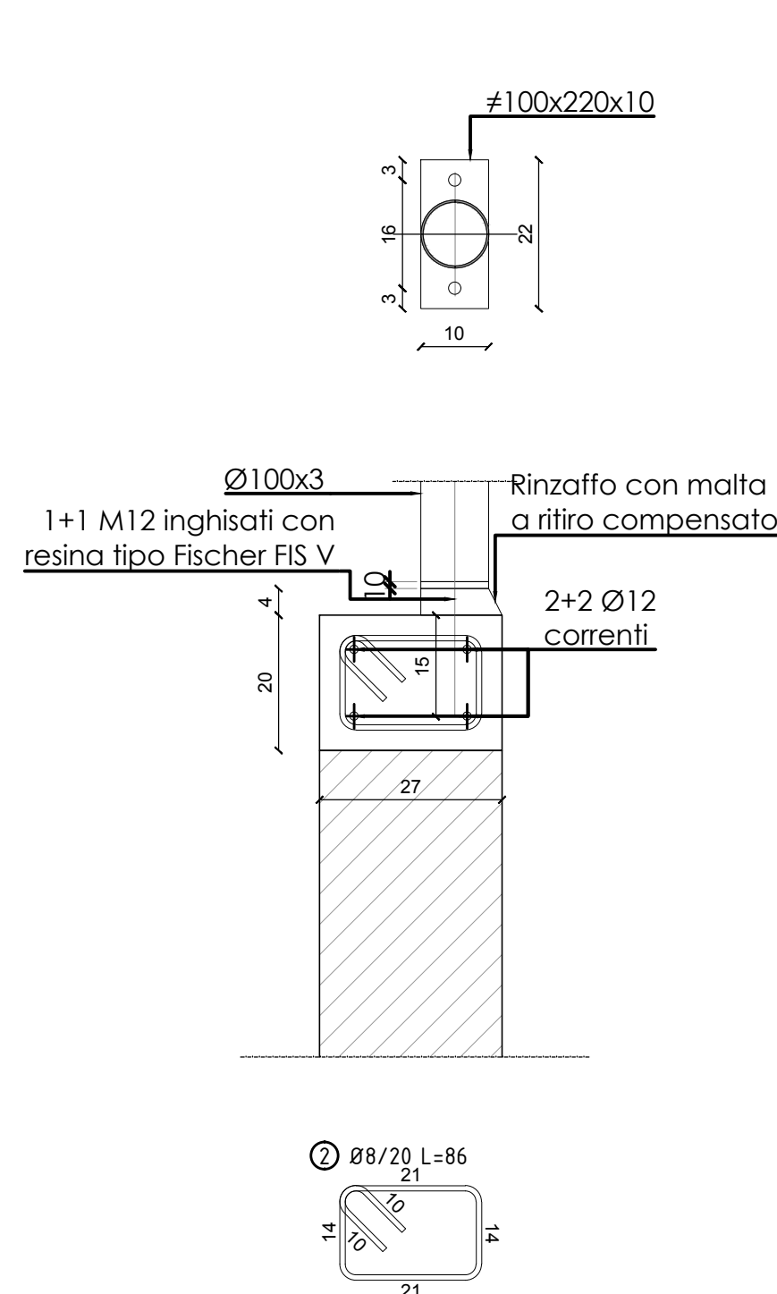
DETTAGLIO F-2 - SCALA 1:10
