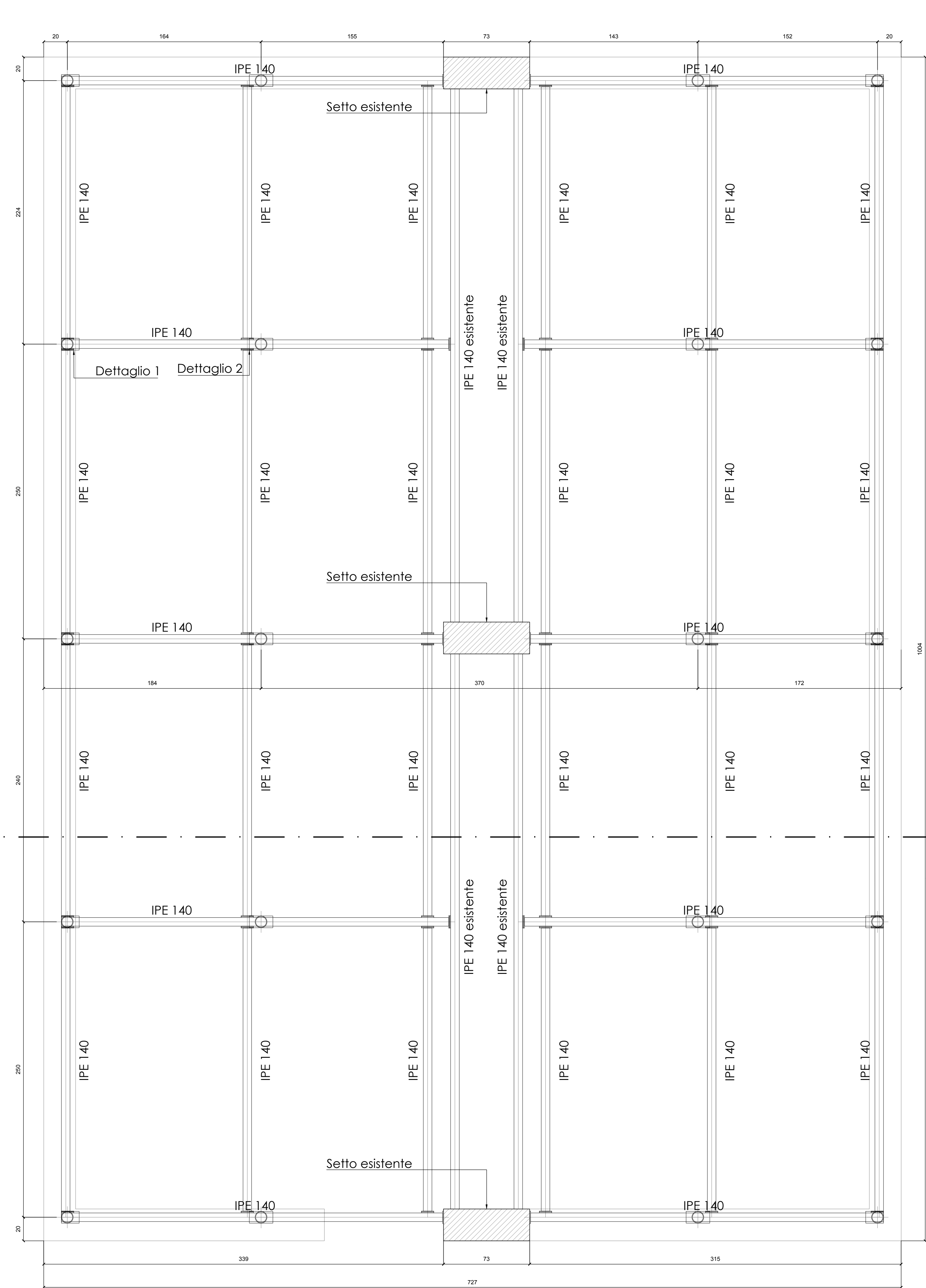
PIANTA - SCALA 1:20
