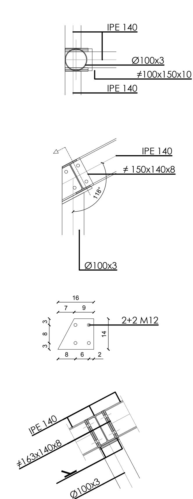
DETTAGLIO 1 - SCALA 1:10
